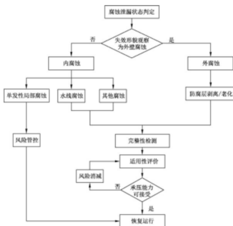
图 3 腐蚀泄漏状态判定流程
