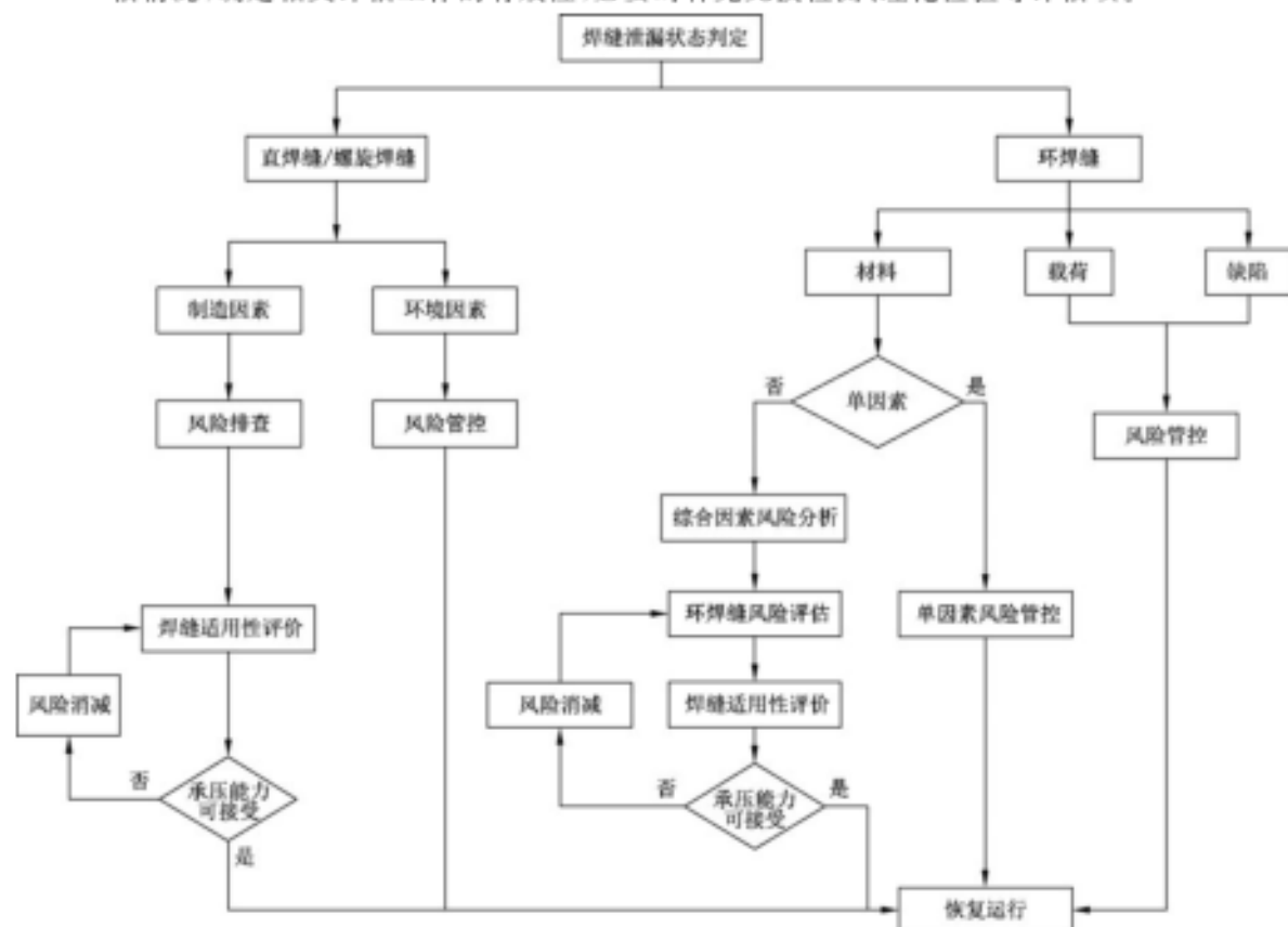
图 2 焊缝泄漏状态判定流程
