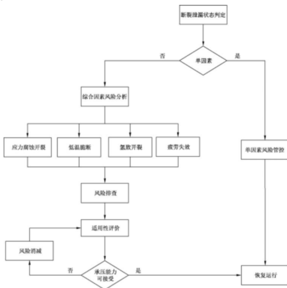
图 4 断裂泄漏状态判定流程
